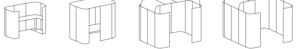
SR/DRHAdjust 201 x 101 x 136 SR/SR 201 x 134 x 191 SR/SMR 268 x 201 x 230 SR/LMR 268 x 268 x 230
